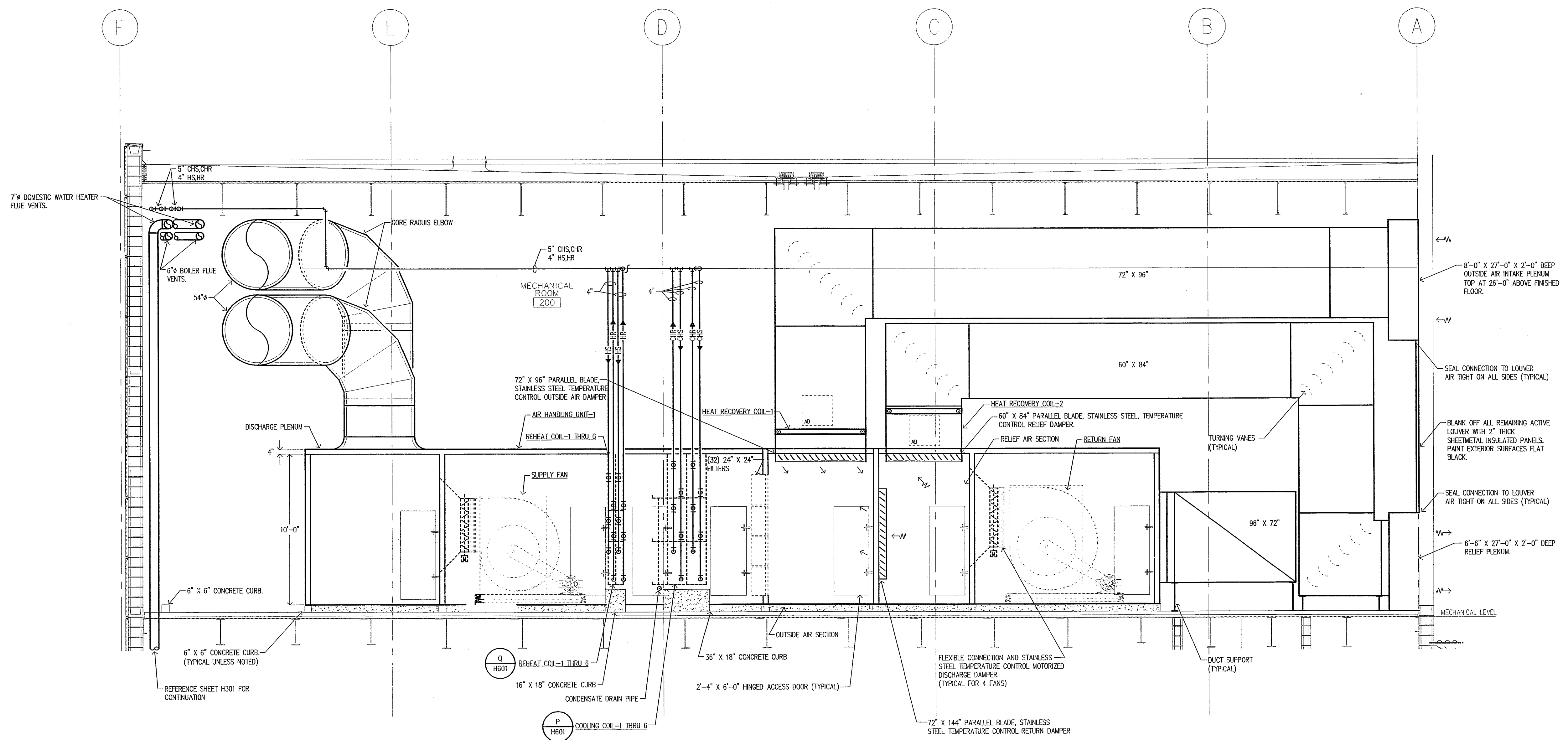
SECTION 1 SCALE: 1/4" = 1'-0"
